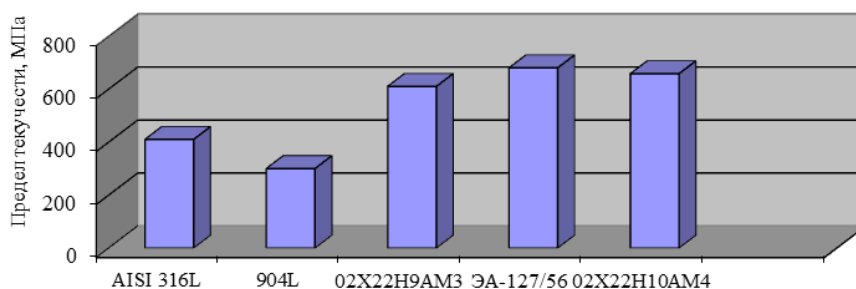
Сравнение предела текучести
