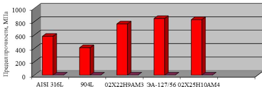
Сравнение предела прочности
